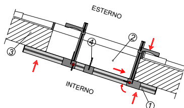
Fig.2 Finestra a tetto
