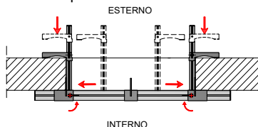
Fig.3 Finestra o porta-finestra
