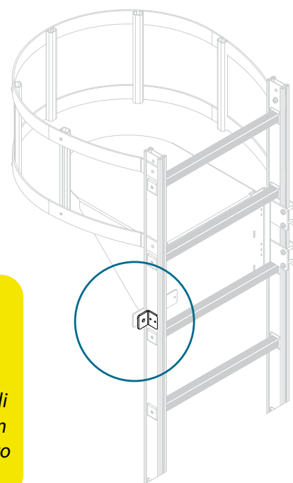
Fig. 16C Fissaggio Battuta Sportello Anti-Intrusione
