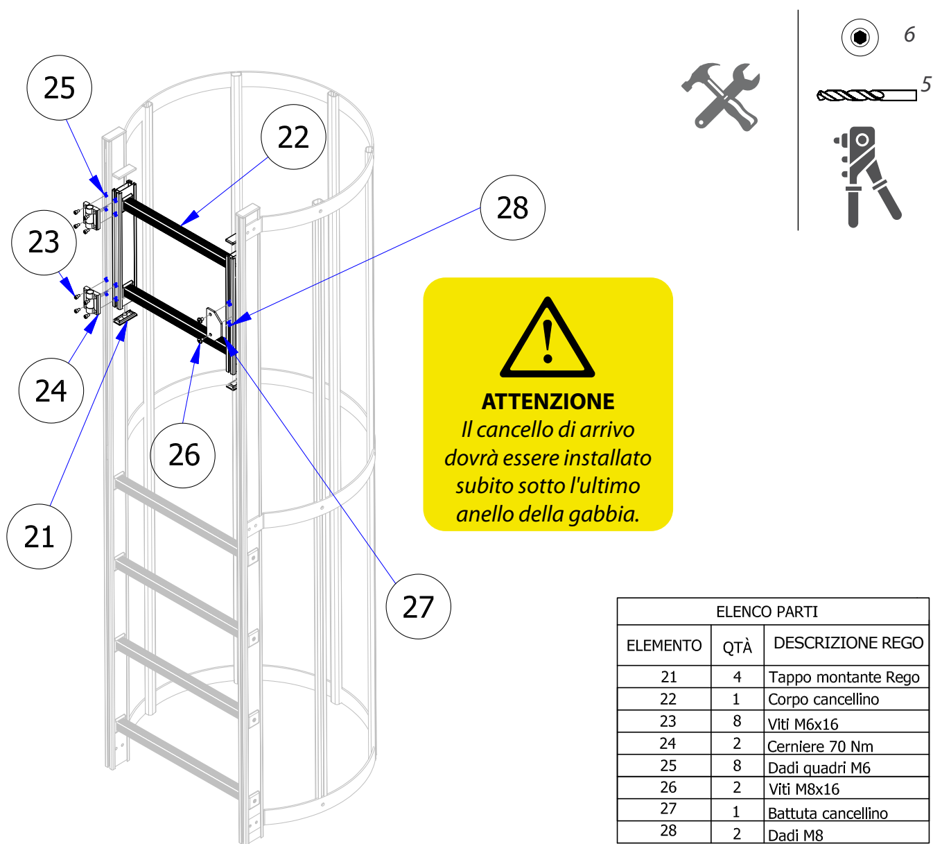
Fig. 11 Fissaggio cancello di arrivo
