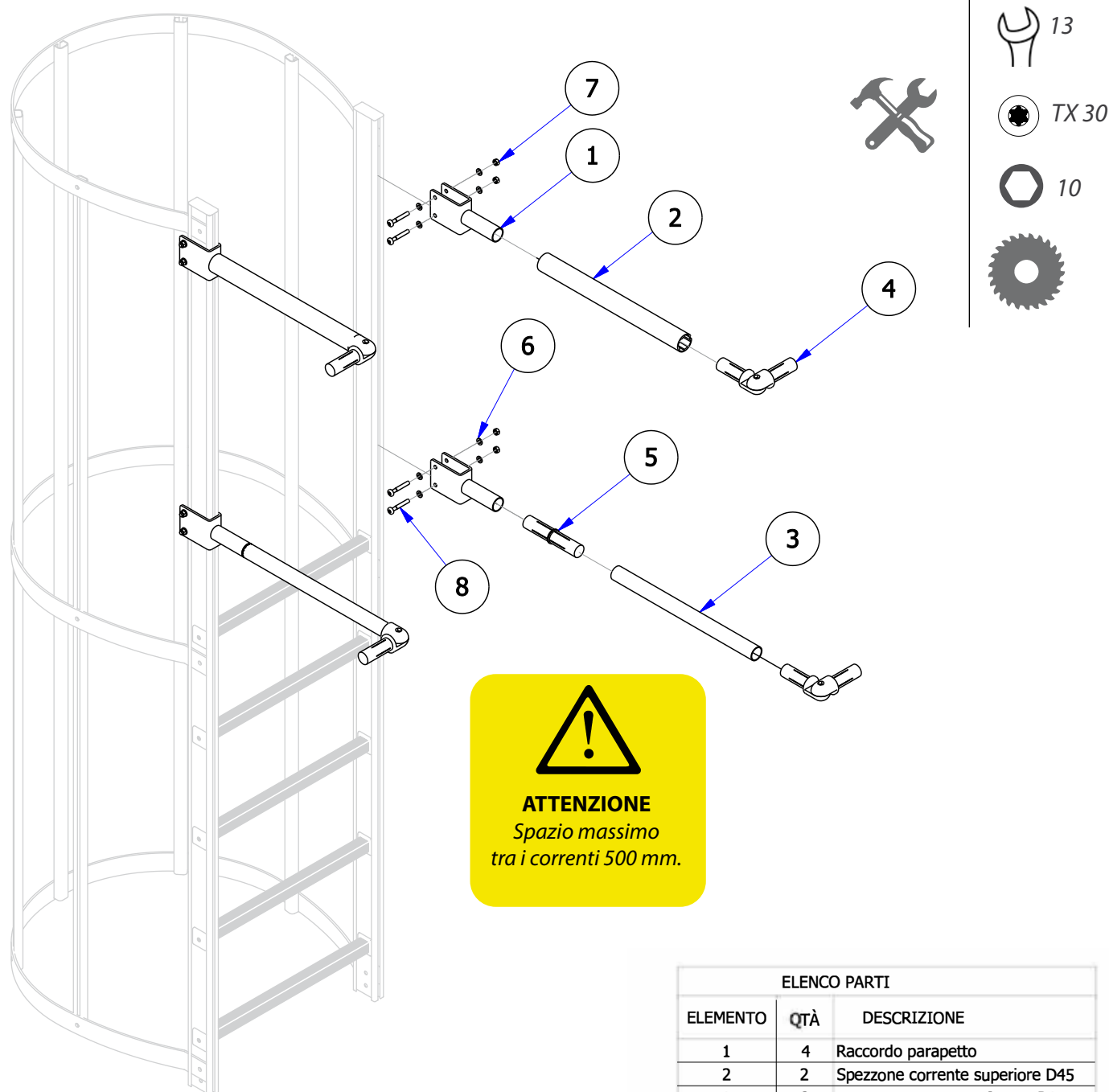
Fig. 18 Assemblaggio raccordo parapetto LIMIT System
