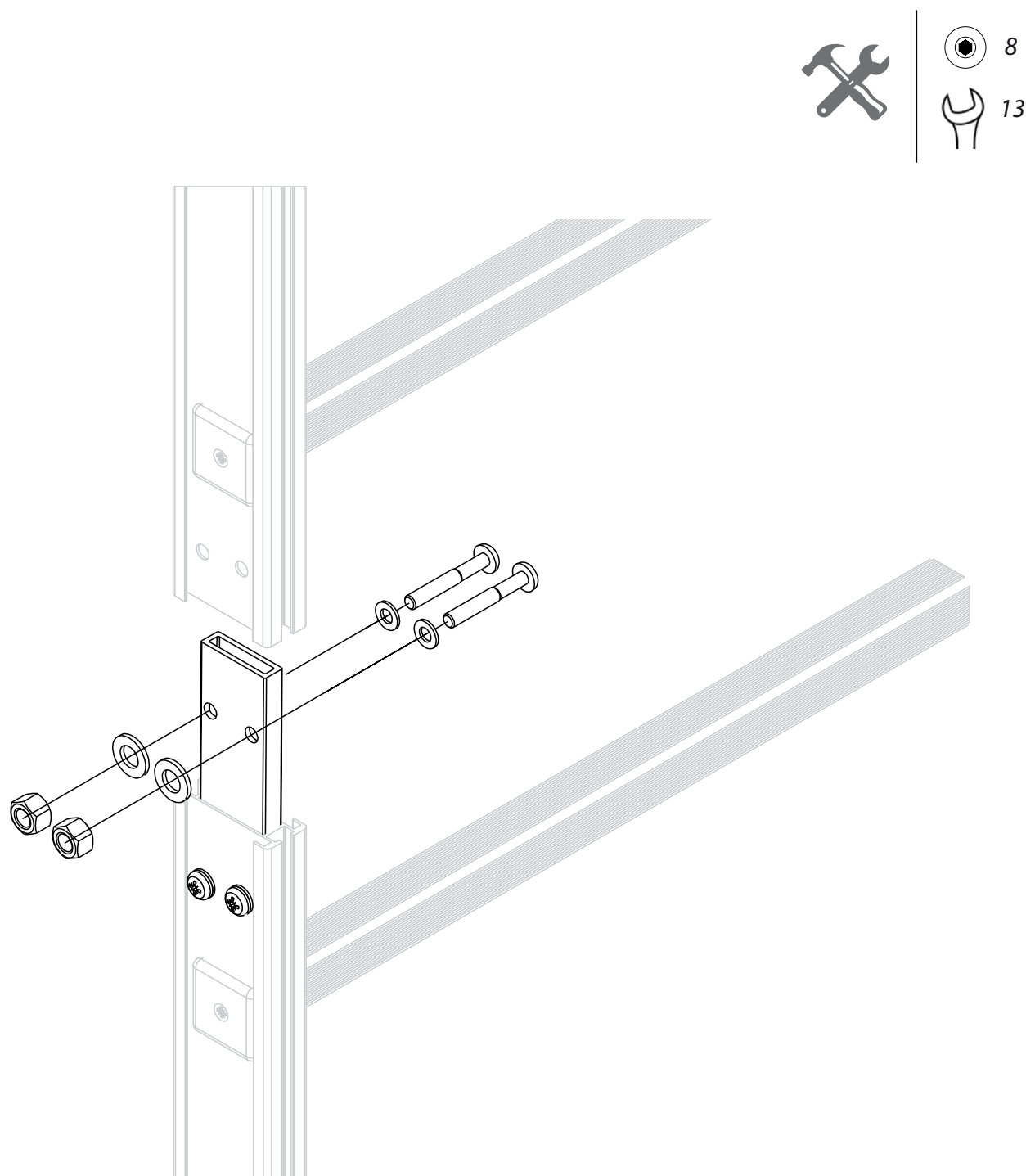
Fig. 3 Collegamento moduli scala
