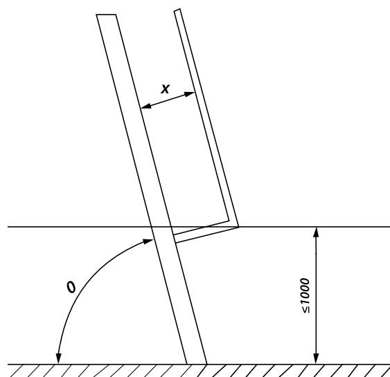
FIG.9 Posizionamento di un corrimano su una scala a castello (Dimensioni in millimetri)
