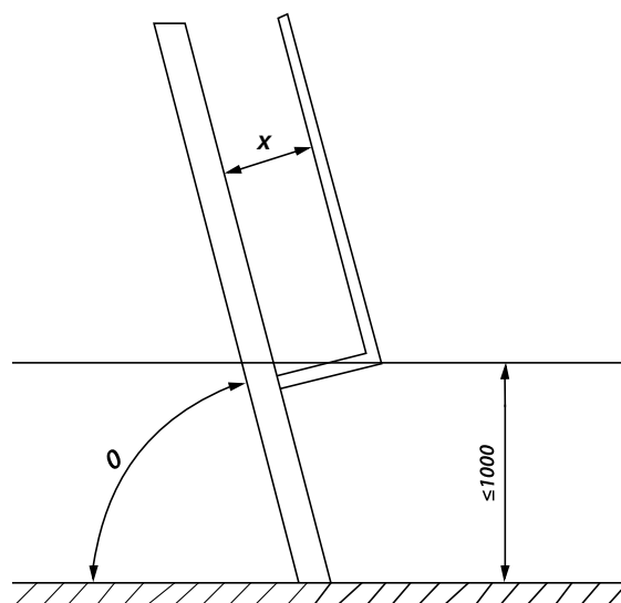
FIG.8 Posizionamento di un corrimano su una scala a castello (Dimensioni in millimetri)
