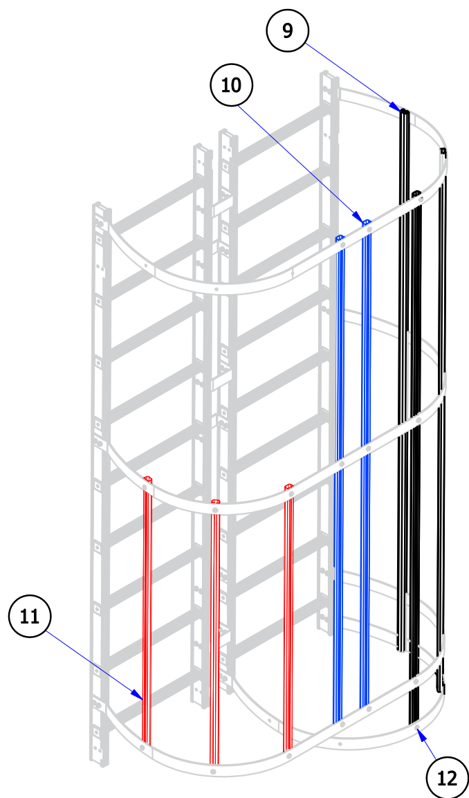
Fig. 20C Fissaggio Profilo Gabbia Modulo Ispezione
