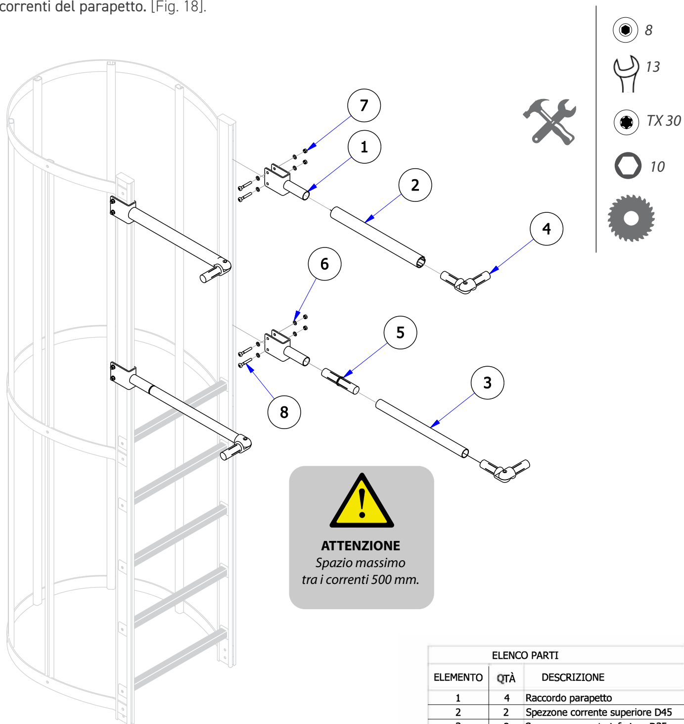
Fig. 18 Assemblaggio raccordo parapetto LIMIT System
