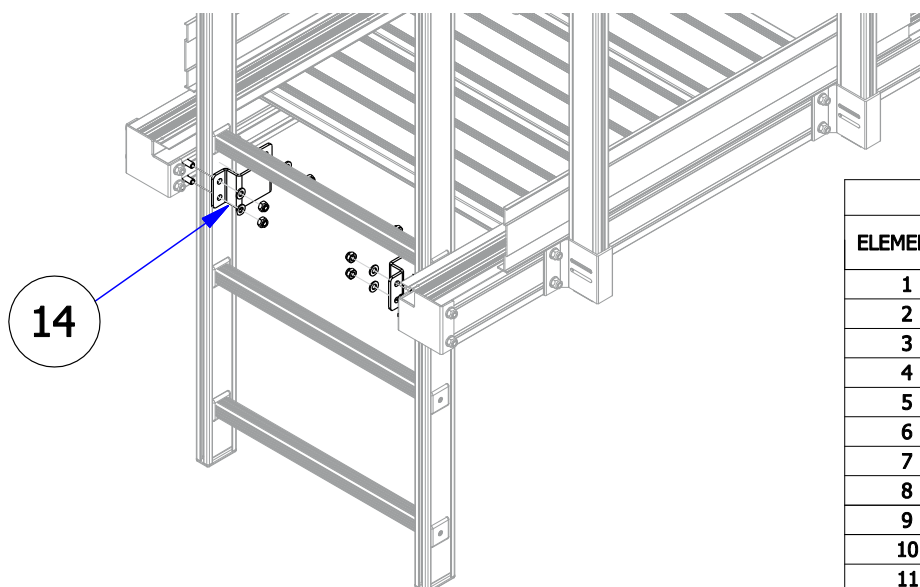
Fig. 24 Collegamento Passerella-Scala
