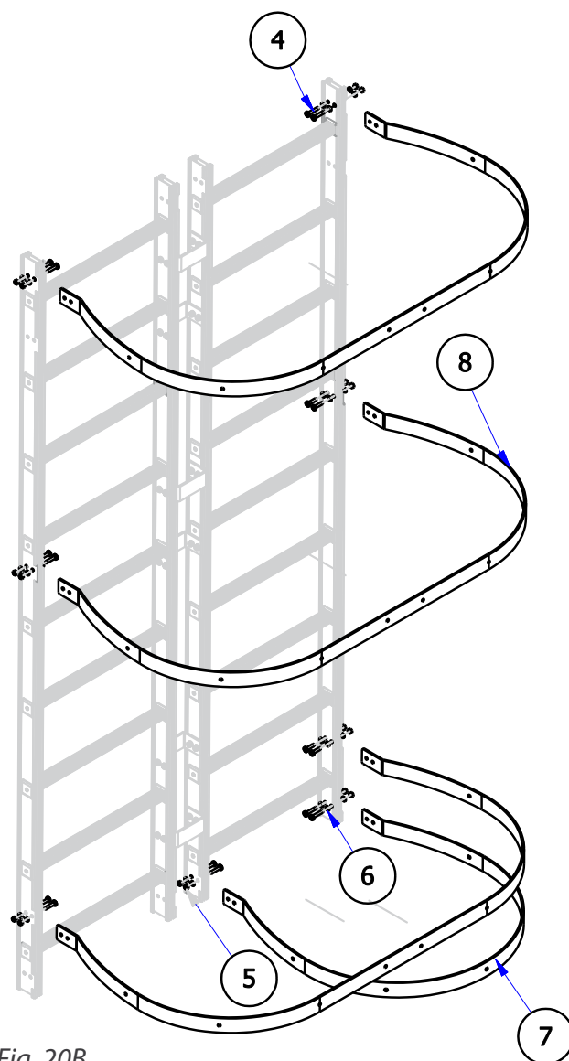
Fig. 20B Fissaggio Anelli Modulo Ispezione
