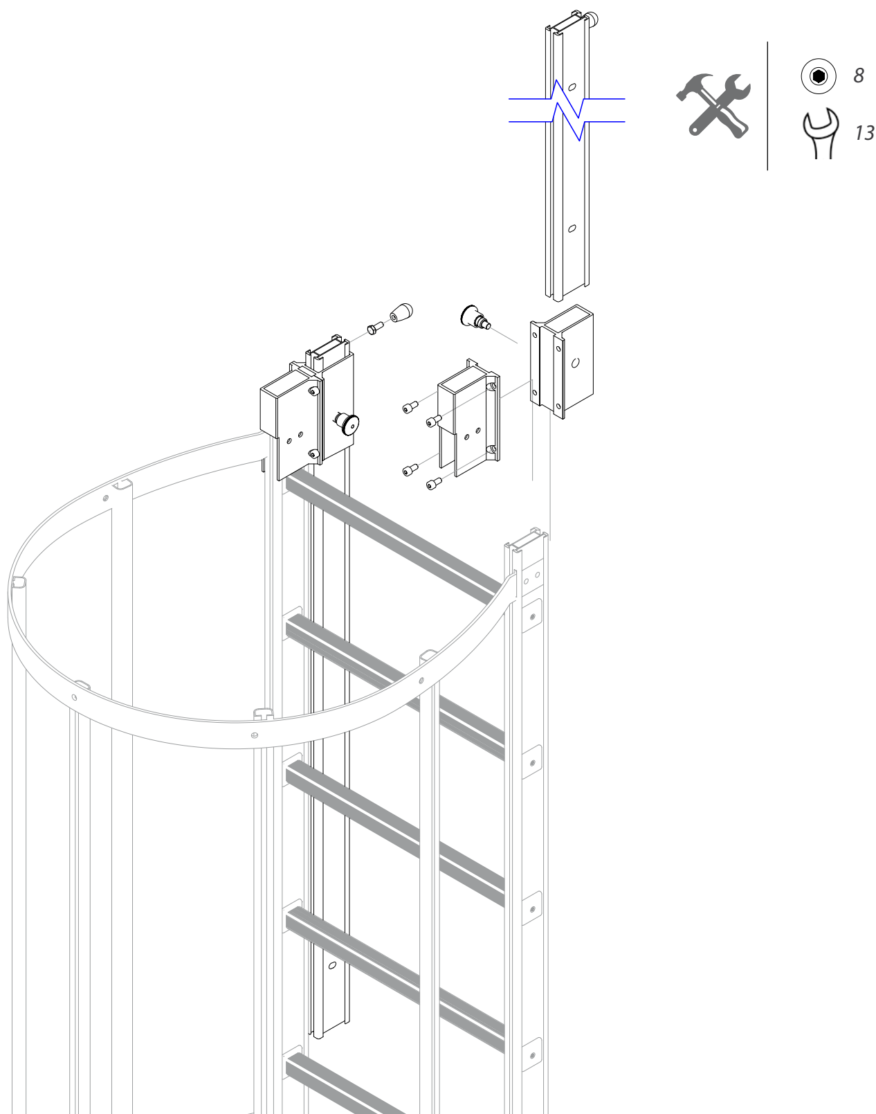
Fig. 22 Fissaggio prolunga montanti estraibili
