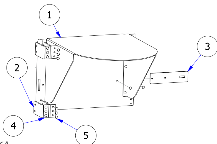
Fig. 16A Assemblaggio elementi Sportello anti-intrusione
