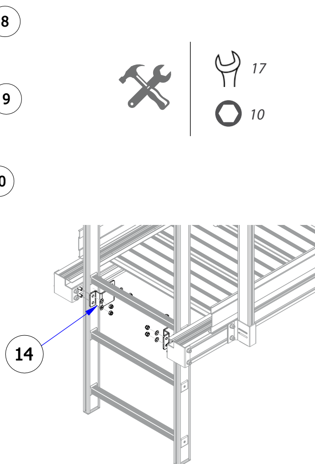
Fig. 26 Collegamento Passerella-Scala
