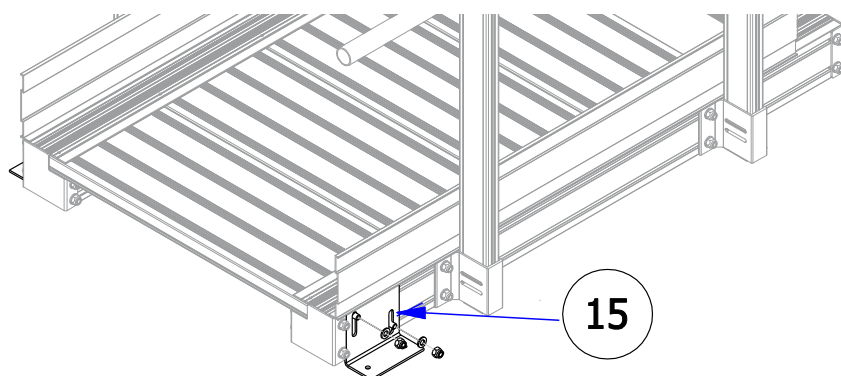
Fig. 27 Installazione L di Fissaggio al Cosciale
