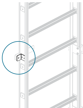
Fig. 15C Fissaggio Battuta Porta Anti-Intrusione
