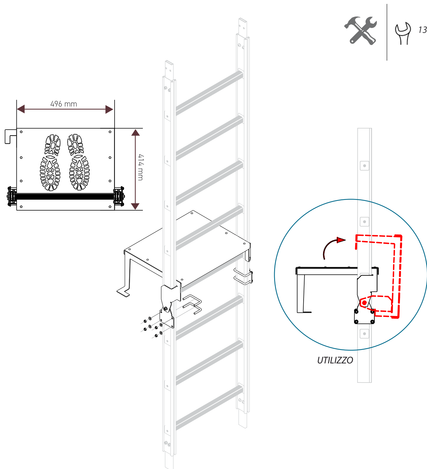
Fig.14 Montaggio piano di riposo ribaltabile
