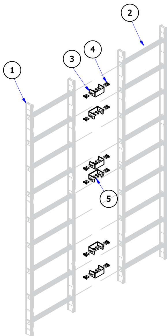
Fig. 19A Assemblaggio elementi giunzione modulo sdoppiamento
