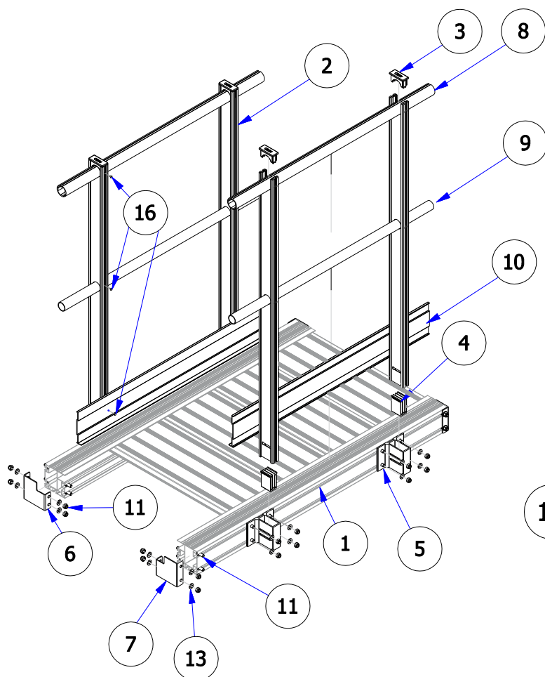
Fig. 25 Installazione Parapetto e Tappi Cosciale
