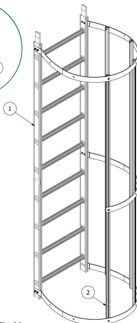
Fig. 30 Uscita laterale assemblata
