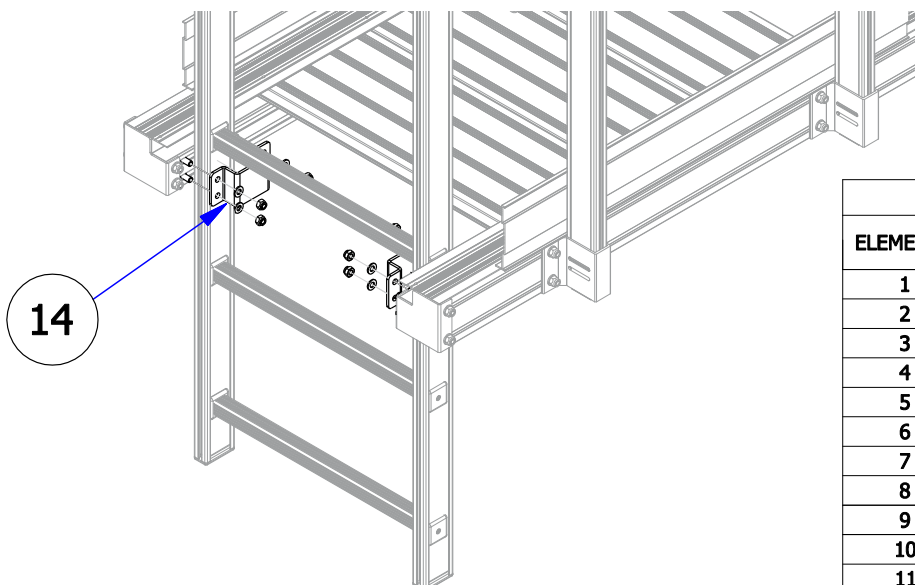
Fig. 23 Collegamento Passerella-Scala
