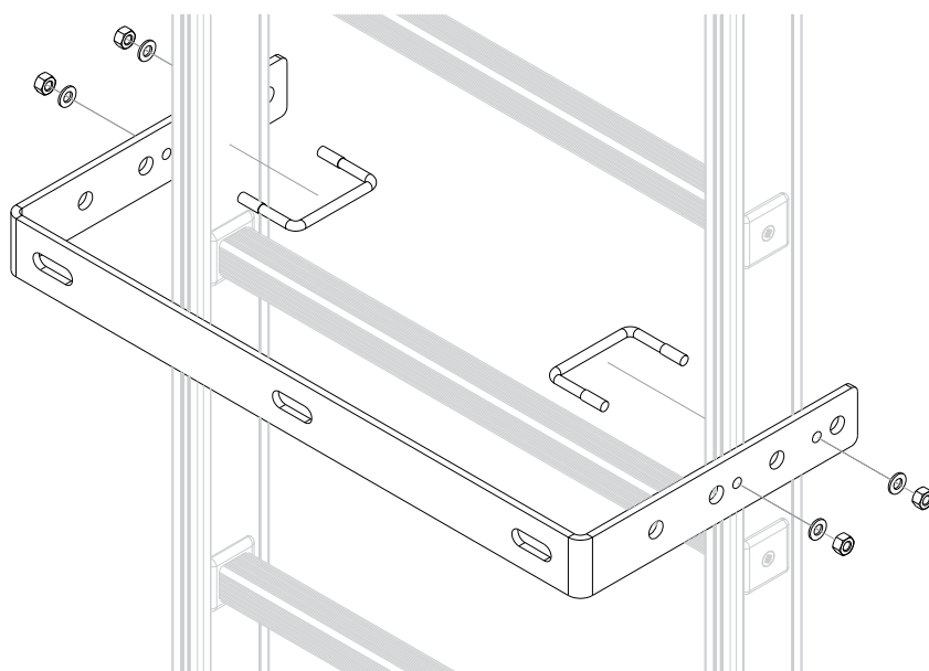
Fig. 7 Fissaggio zanca unica 180mm
