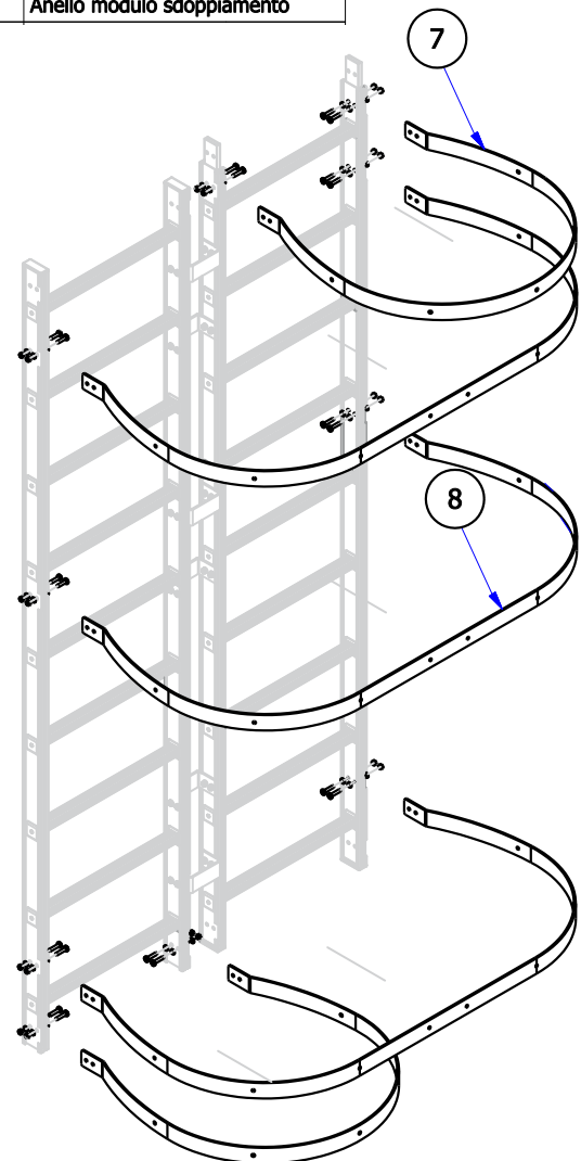
Fig. 19B Fissaggio Anelli Modulo Sdoppiamento
