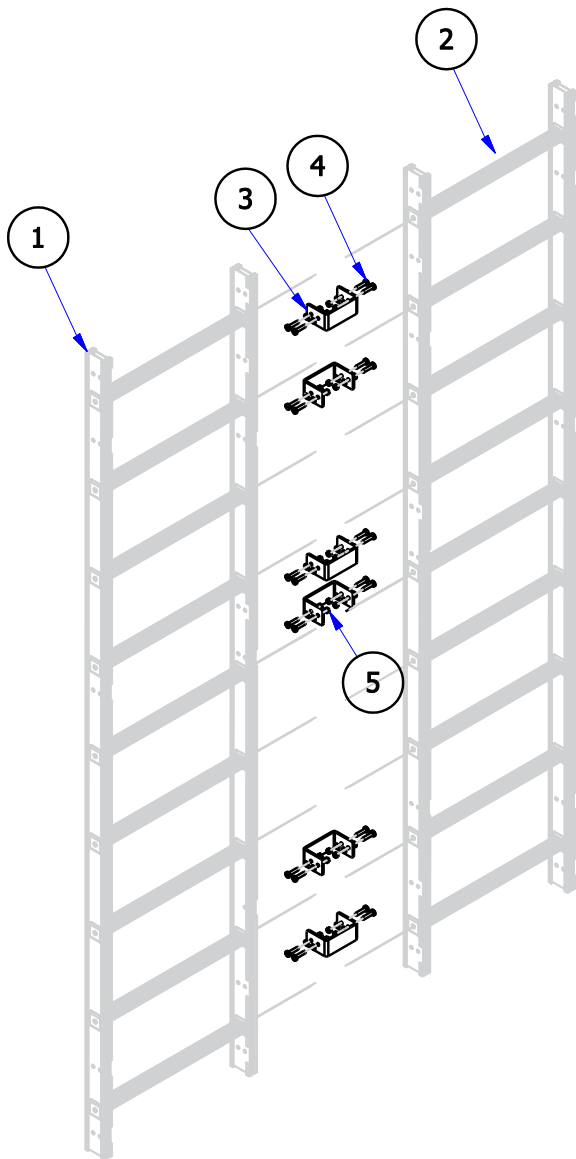
Fig. 19A Assemblaggio elementi giunzione modulo sdoppiamento
