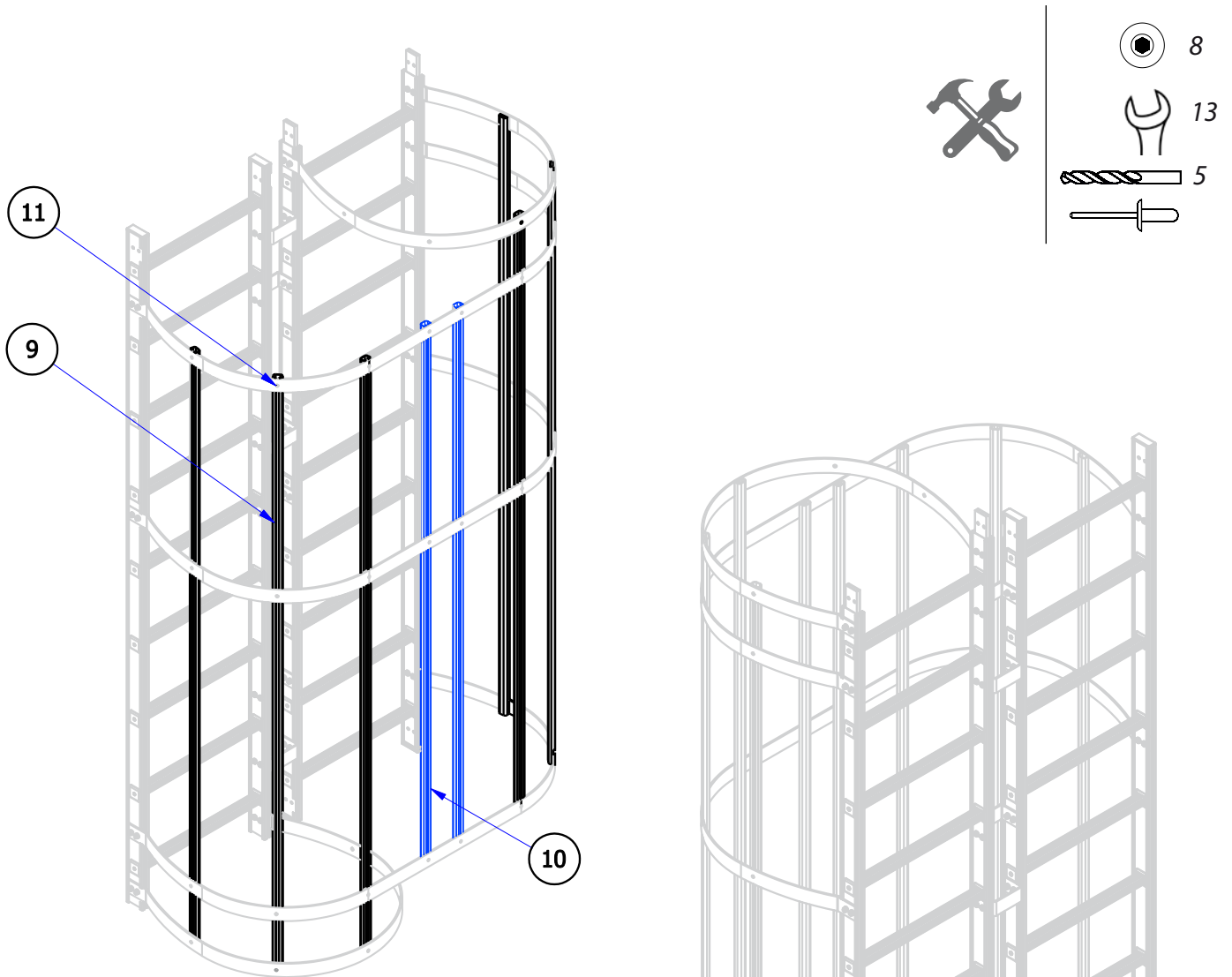
Fig. 19C Fissaggio Profilo Gabbia Modulo Sdoppiamento
