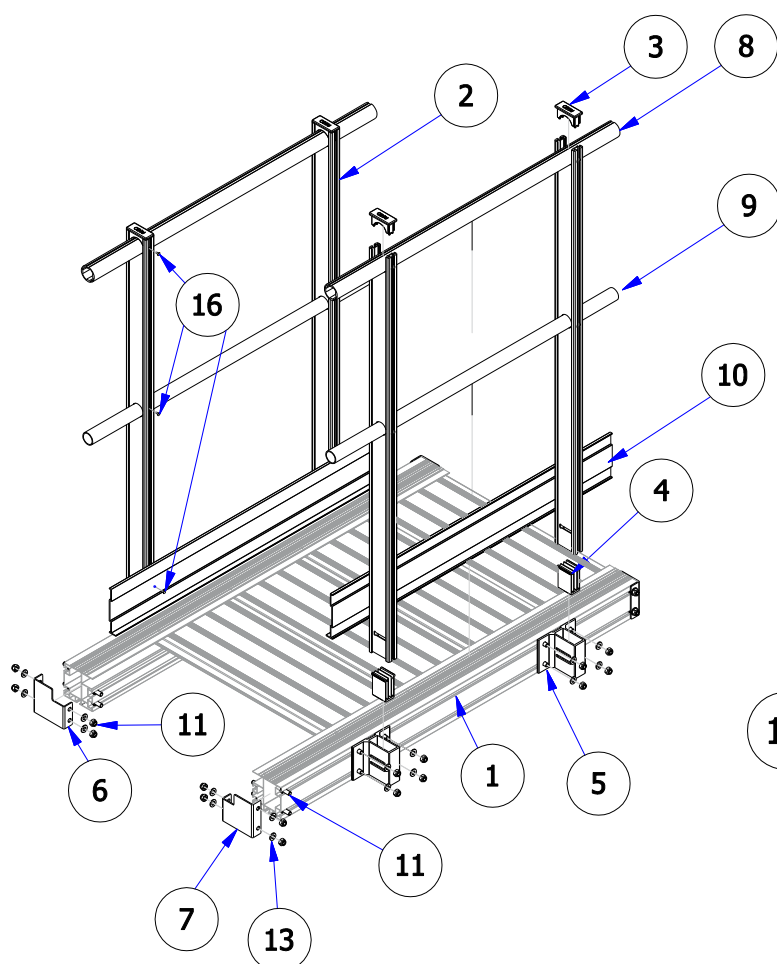
Fig. 24 Installazione Parapetto e Tappi Cosciale
