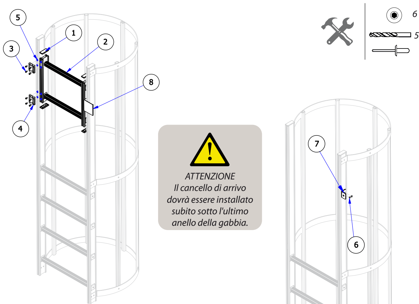
Fig. 11 Fissaggio cancello di arrivo
