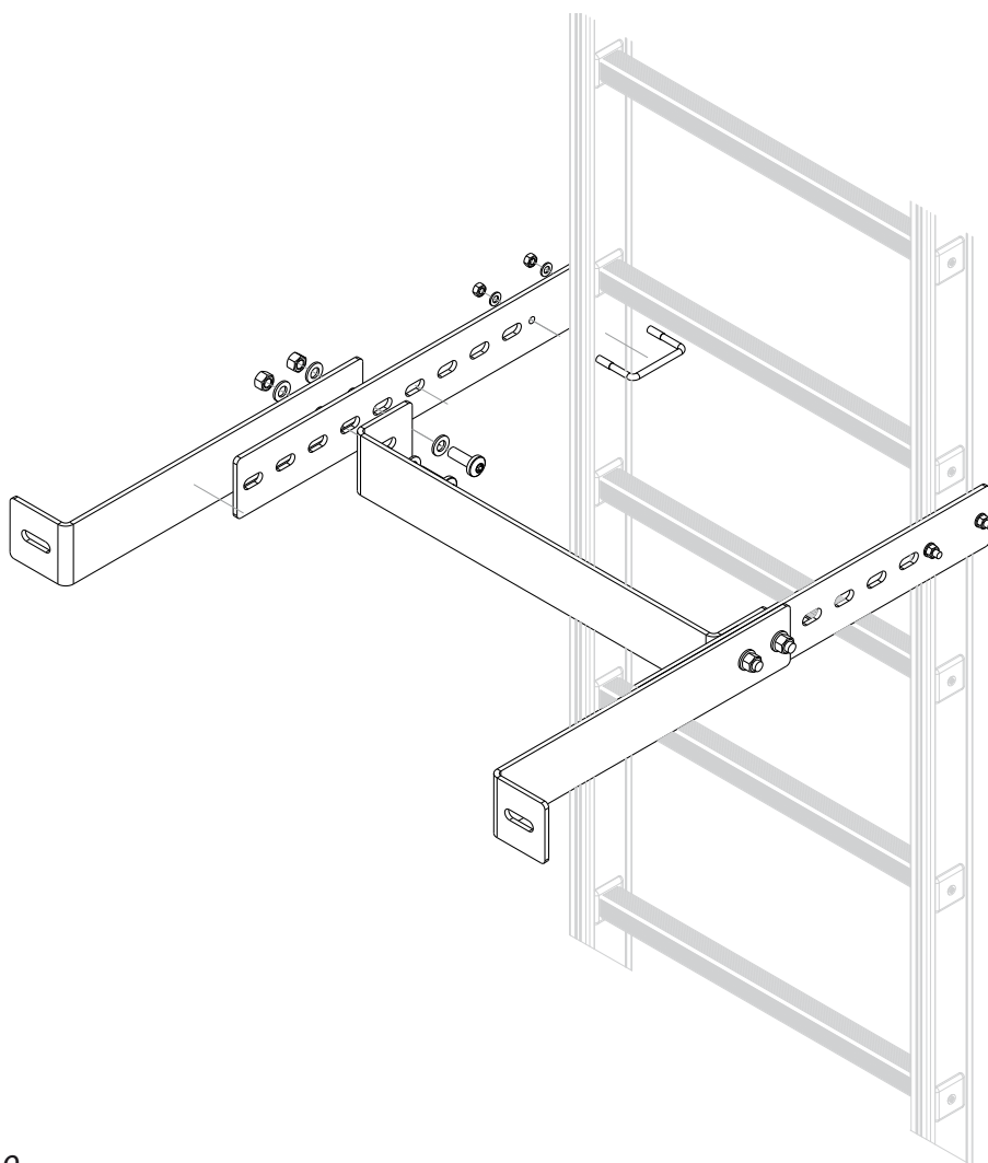
Fig. 9 Fissaggio zanca con prolunga 450-800mm
