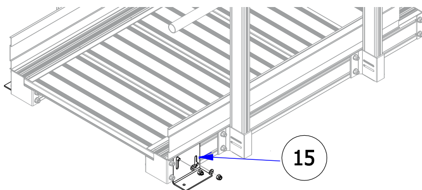
Fig. 26 Installazione L di Fissaggio al Cosciale
