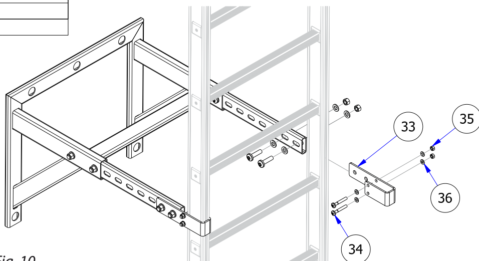
Fig. 10 Fissaggio zanca tralicciata
