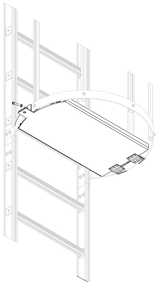
Fig. 17C Fissaggio Battuta Botola Anti-Intrusione
