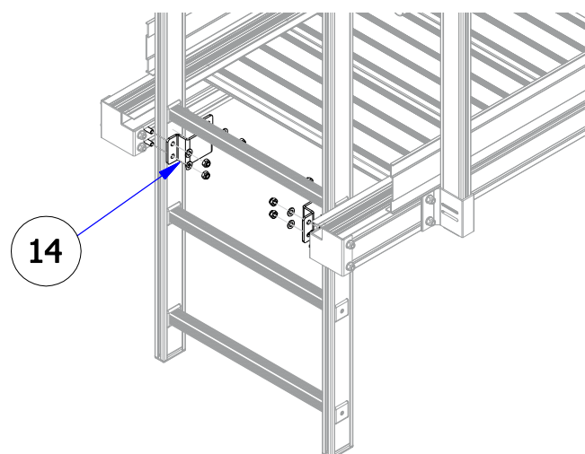
Fig. 25 Collegamento Passerella-Scala
