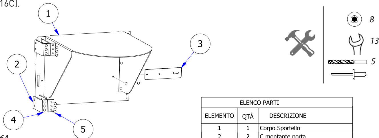
Fig. 16A Assemblaggio elementi Sportello anti-intrusione
